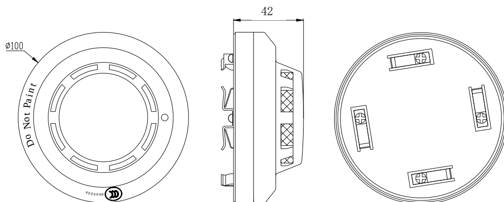
图 1 探测器外形示意图
