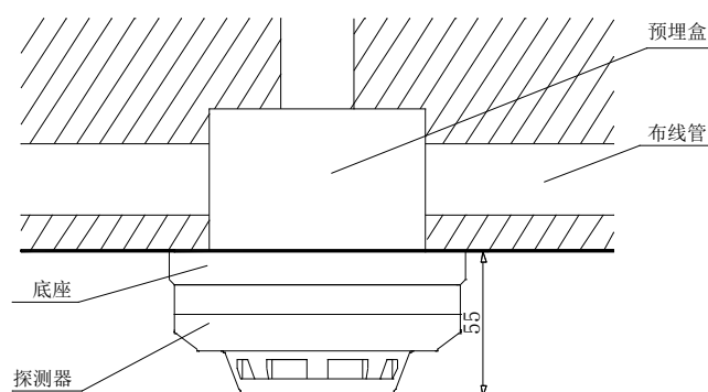
图 2 探测器安装示意图
