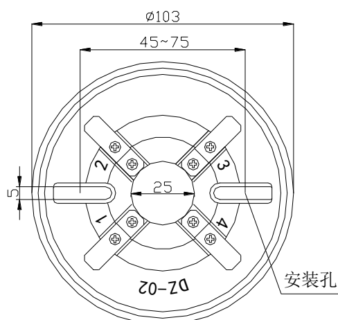
图 3 探测器通用底座外形示意图
