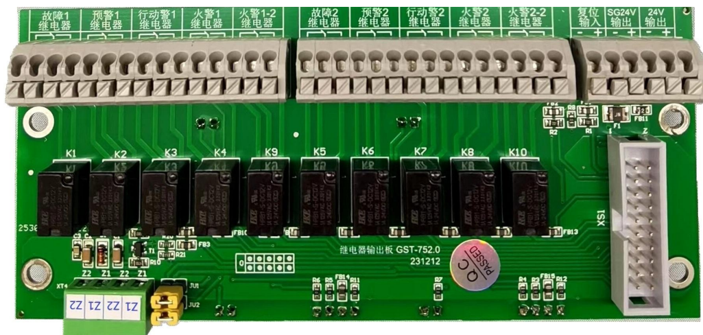
图 4.3 继电器板与外部连接示意
