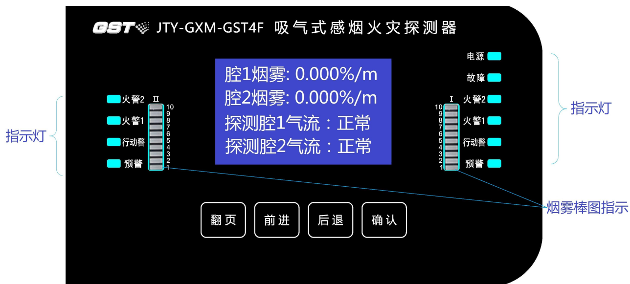
图 2.2 显示操作面板说明
